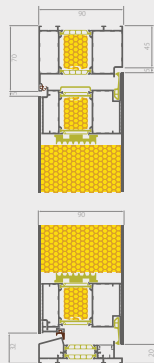
Coupe du cadre de la porte d'épaisseur de 90 mm et d'un battant de porte d'épaisseur de 90 mm
